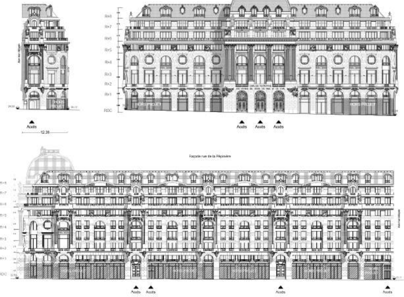
Façade rue Labordé
